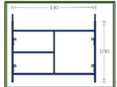
Andamio Enano
