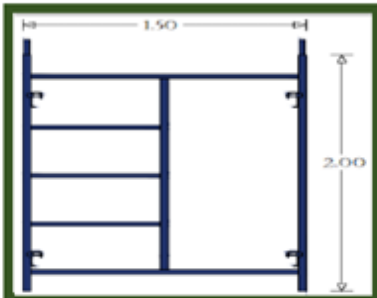
Andamio Estándar
