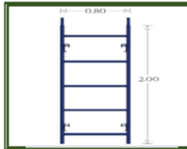
Andamio Angosto
